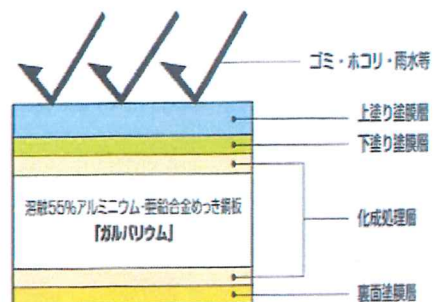
<スラット断面>
